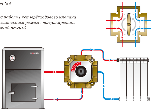
Схема №4
