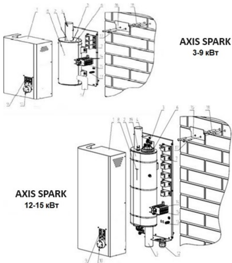
Рис.1 Конструкция котла
