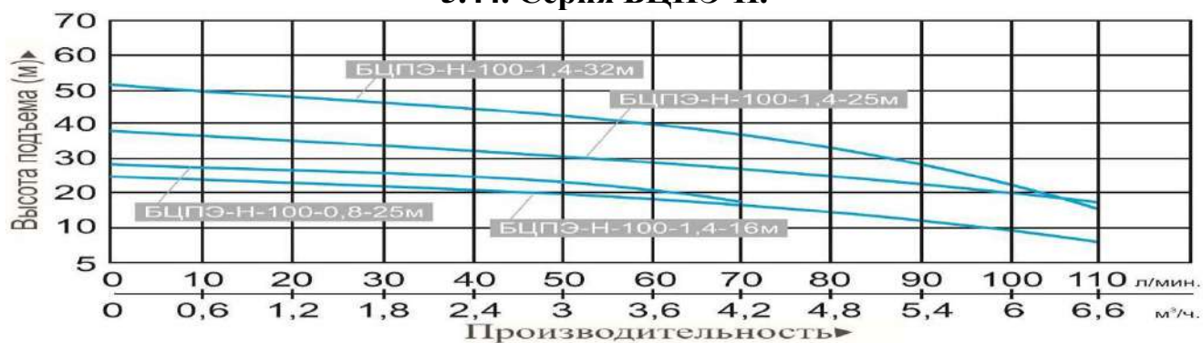
5.45. Серия БЦПЭ-100/150.
